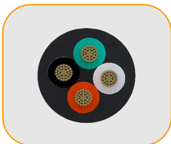
Corte Transversal
